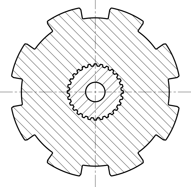
Ж-Ж (1:1) Парковочный тормоз
